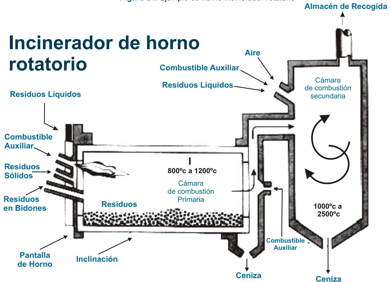
Figura 24. Ejemplo de horno incinerador rotatorio
